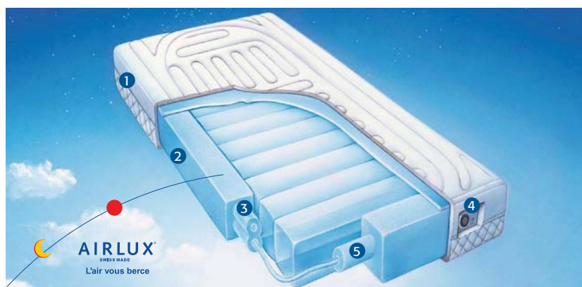
AIRLUX® matelas à air avec 1 Revêtement isolant 2 Cadre de mousse 3 Pompe à cœur souple 4 Mollette de réglage de la fermeture 5 Réservoir
